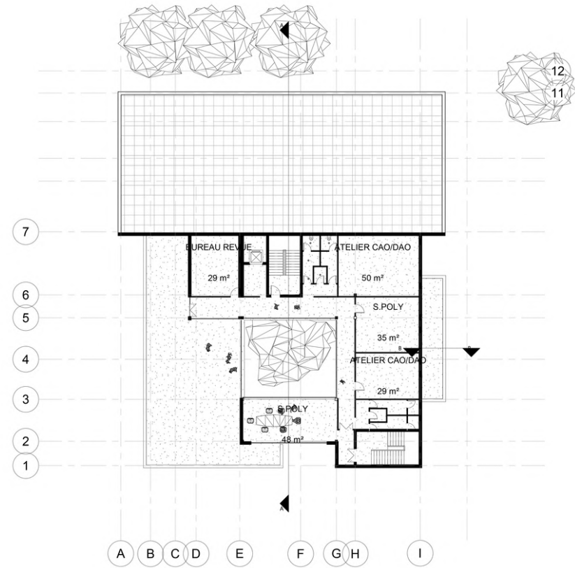
Niveau 4 1 : 200
