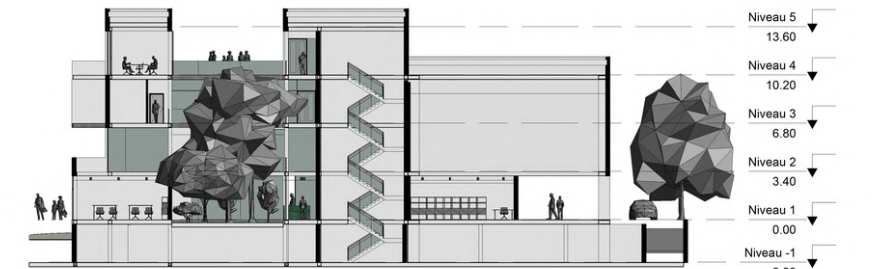
A 1 : 200
