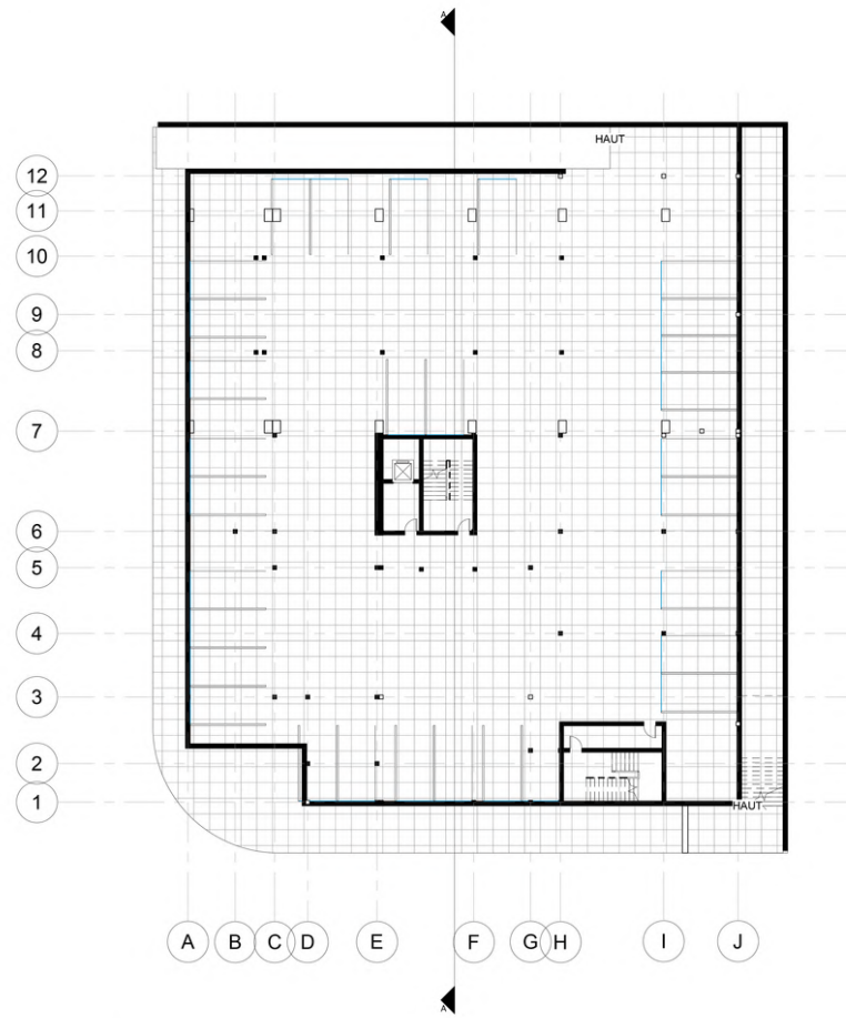
Niveau -1 1 : 200
