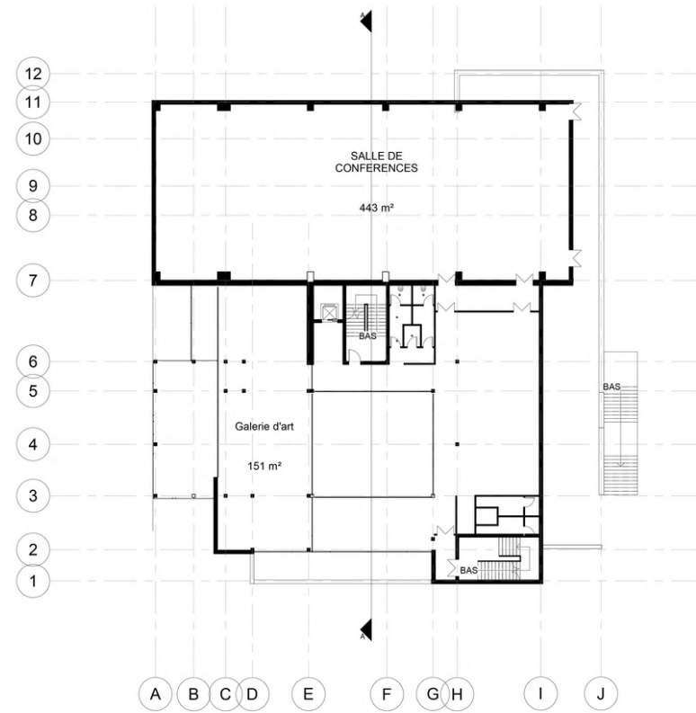
Niveau 2 1 : 200
