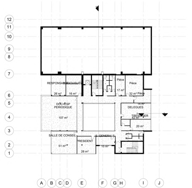
Niveau 3 1 : 200
